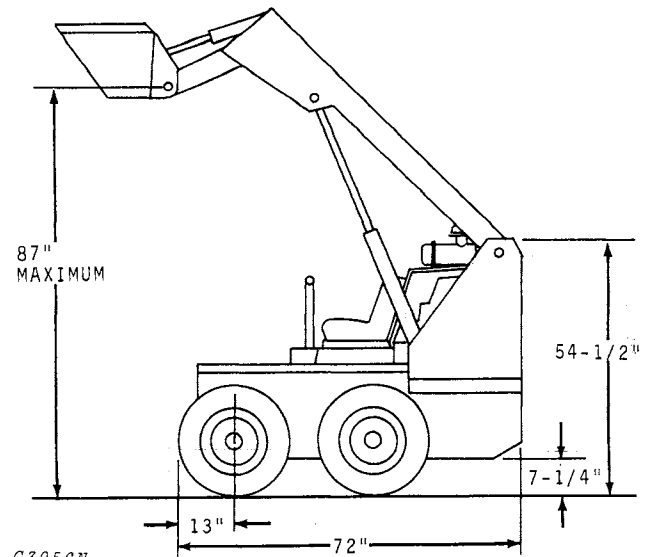
Fig. 3-Loader Dimensions
